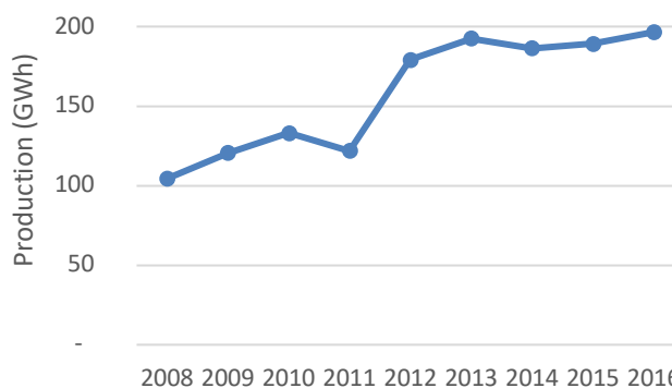
Figure 9 : Évolution de la production d'EnR&R selon les années Source : Outil BASEMIS, Air Pays de la Loire
