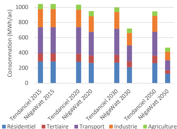
Figure 10 : Potentiel de réduction de consommation énergétique
