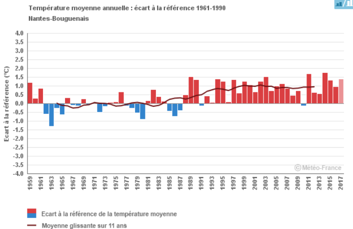
Figure 14 : Évolution des températures moyennes annuelles à Nantes – Bouguenais depuis 1959, Source : Météo France – Climat HD
