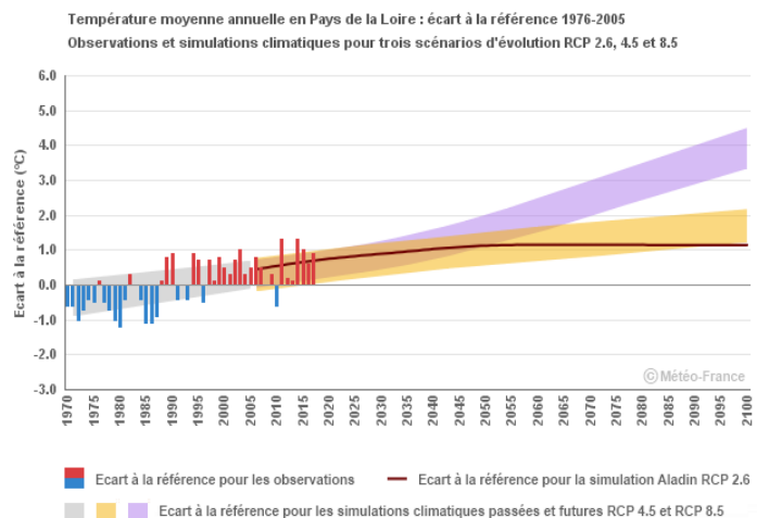
Figure 15 : Évolution des températures moyennes annuelles en région Pays de la Loire, source : Météo France – Climat HD
