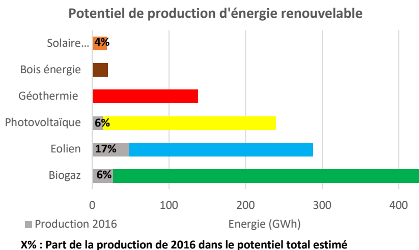
Figure 11 : Potentiel de production d'énergie renouvelable
